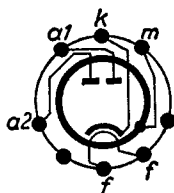
Sockelschaltschema
